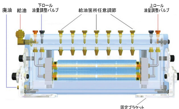
TO-FA型(ロール径φ32mm) TO-FB型(ロール径φ22mm) ※フェルトロール摩耗後交換
